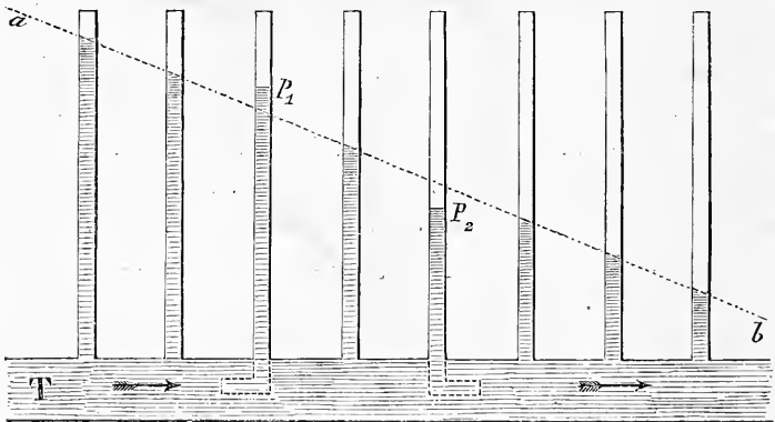
Fig. 143. — Tube T dans lequel se fait un écoulement de liquide dans le sens des flèches a , b , niveaux d'une série de piézomètres. — P 1 et P 2 , tubes de Pitot, diversement orientés; leurs niveaux diffèrent de ceux des piézomètres.
